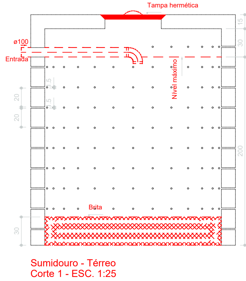
Sumidouro - Térreo Corte 1 - ESC. 1:25
