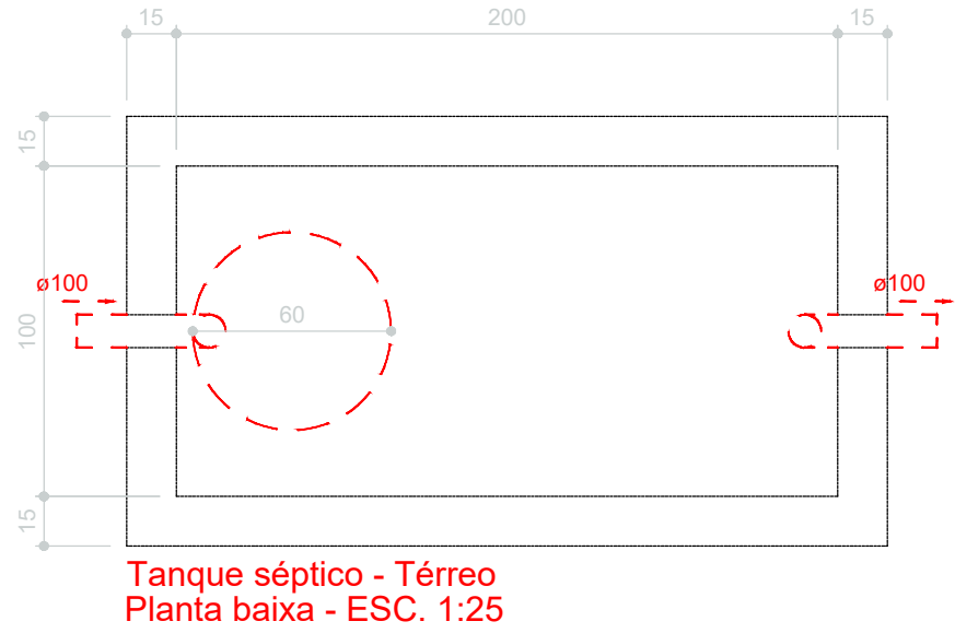
Tanque séptico - Térreo Planta baixa - ESC. 1:25
