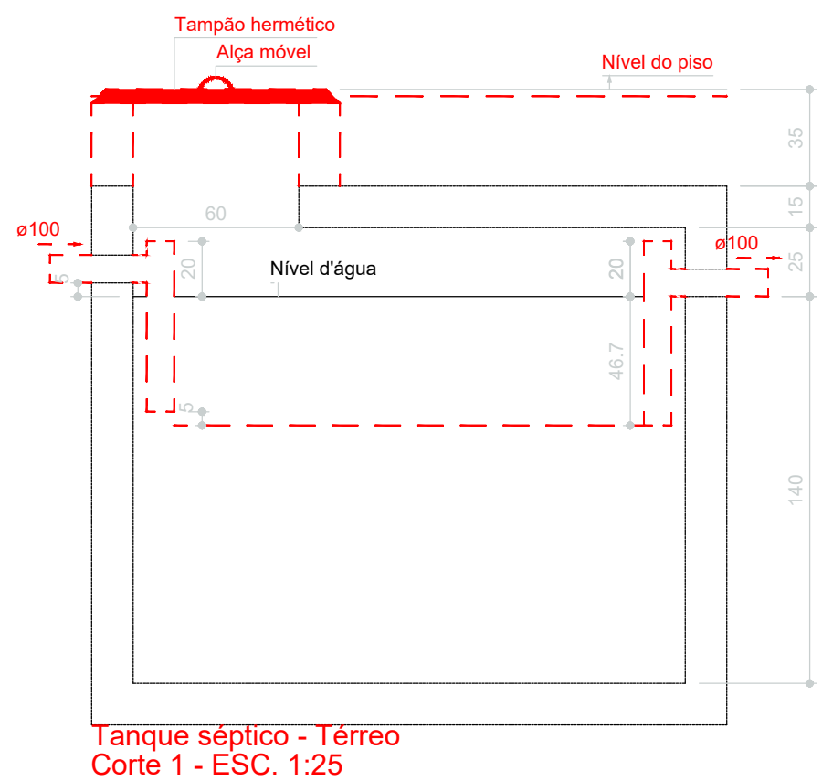
Tanque séptico - Térreo Corte 1 - ESC. 1:25
